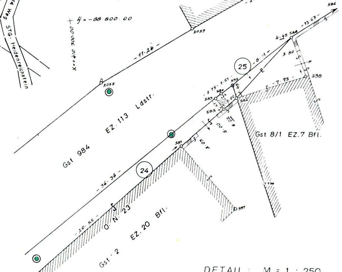
DETAIL: M = 1 : 250
