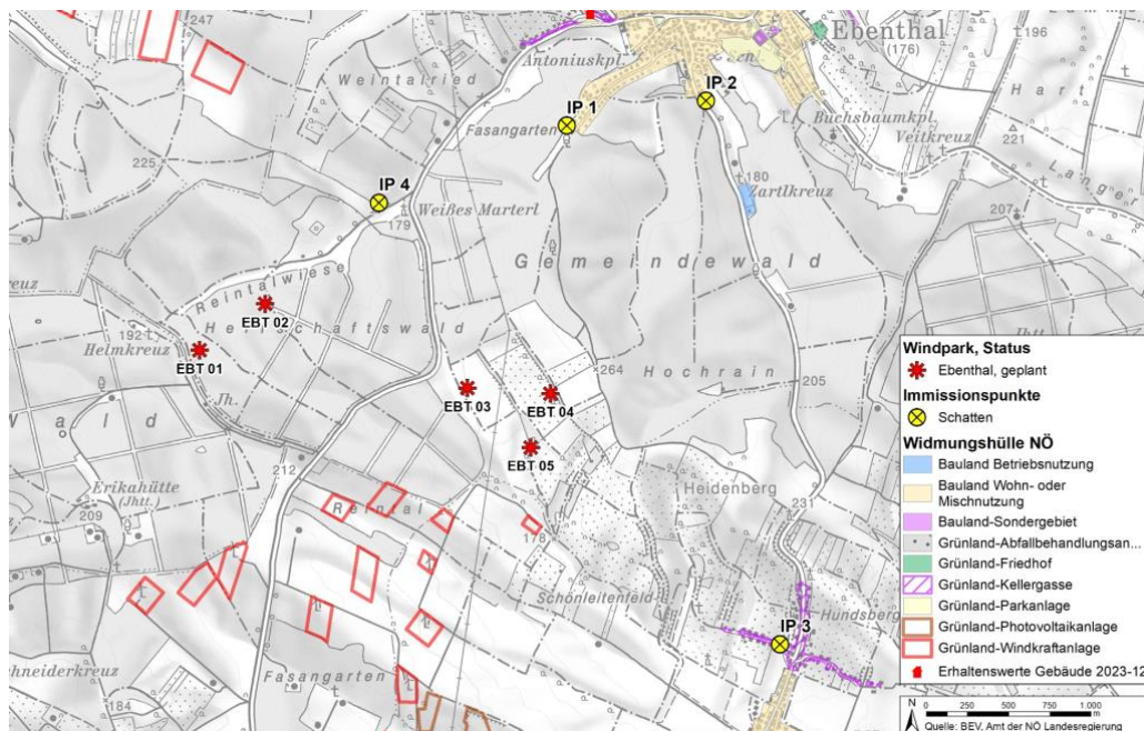
Betrachtete Immissionspunkte beim Schattenwurf
