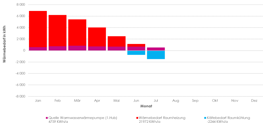
Grafik 63: Wärme- und Kältebedarf, Haus 2
