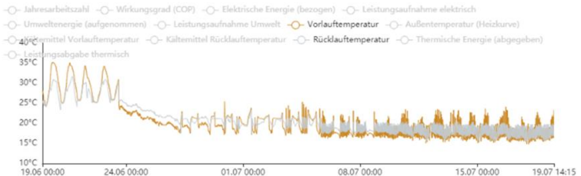
Grafik 68: Vorlauf- und Rücklauftemperatur der Wärmepumpe während der Inbetriebnahme der Kühlung
