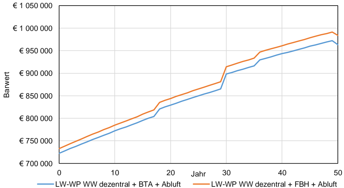
Grafik 35: Vergleich Fußbodenheizung und Bauteilaktivierung
