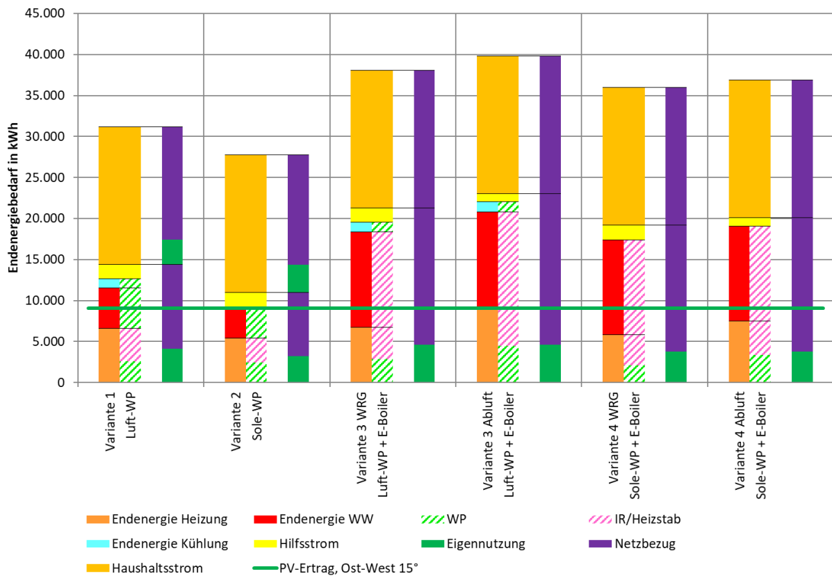
Grafik 29: Variantenberechnung
