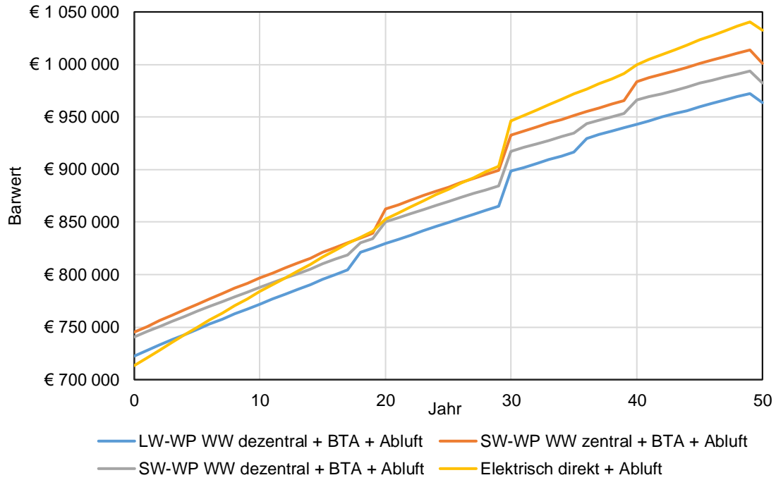
Grafik 34: Vergleich der Haustechnikvarianten mit Wärmeübertragung durch Bauteilaktivierung
