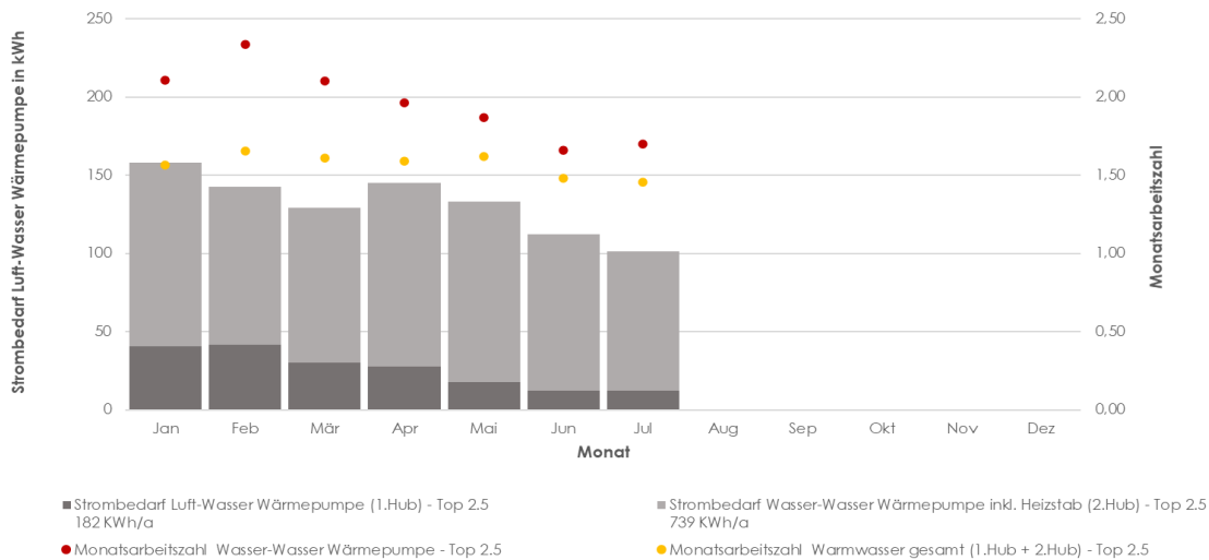
Grafik 71: Strombedarf Wasser-Wasser Wärmepumpe und Monatsarbeitszahl (Top 2.5)
