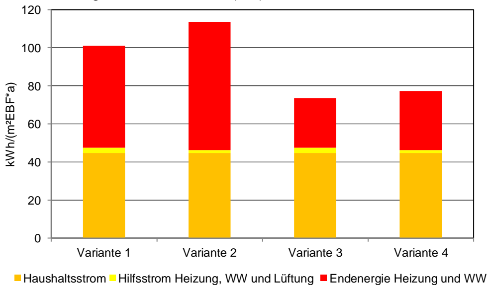
Grafik 27: Variantenvergleich: 23°C und 22,4l/(P*d)
