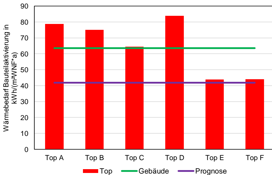
Grafik 38: Wärmebedarf Bauteilaktivierung pro Top und Gebäude im Vergleich zu Prognose
