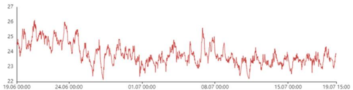
Grafik 69: Raumlufthtemperatur Wohnküche (Top 2.3) während der Inbetriebnahme der Kühlung
