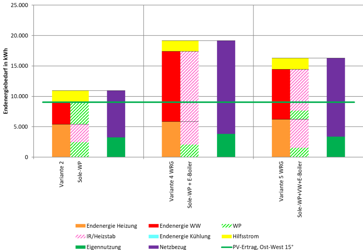
Grafik 30: Variantenberechnung
