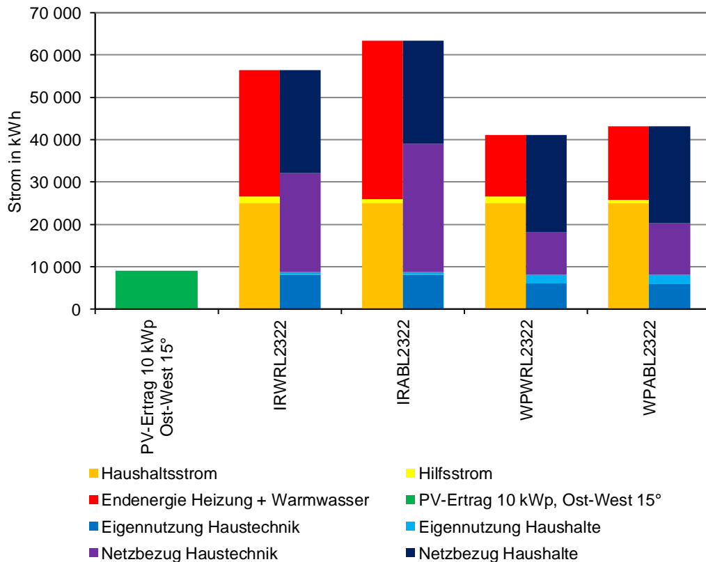
Grafik 28: Stromaufbringung und -verbrauch
