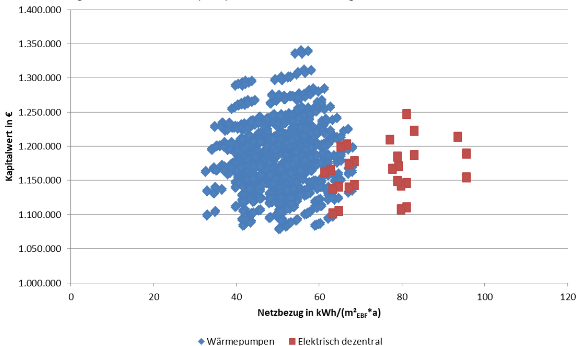
Grafik 33: Ergebniswolke Wärmepumpe vs. Infrarotheizung
