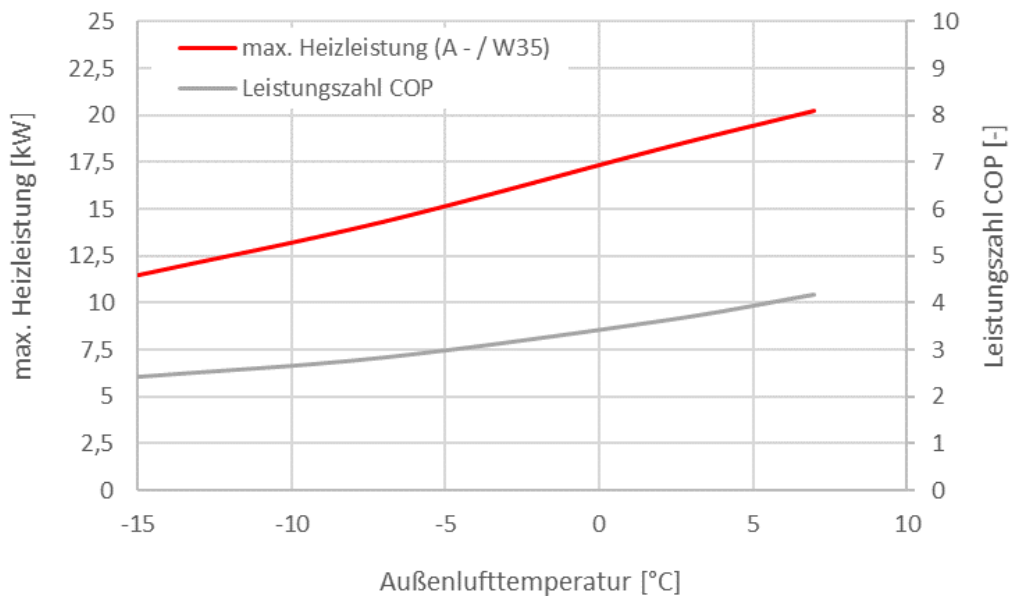
Grafik 59: Heizleistung und Leistungszahl der Luft-Wasser Wärmepumpe in Abhängigkeit der Temperatur auf der Quellenseite [Ovum]
