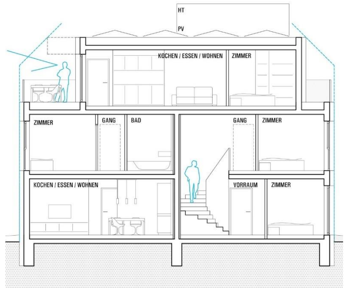
Schnitt
