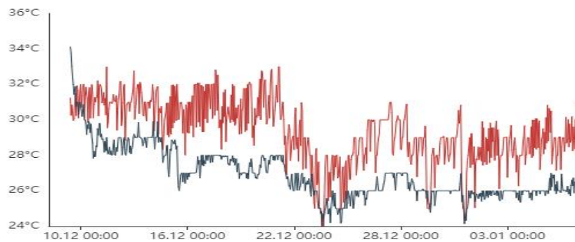
Grafik 66: Vorlauf- und Rücklauf-temperatur am Heizkreisverteiler (Top 2.5) während der Inbetriebnahmephase
