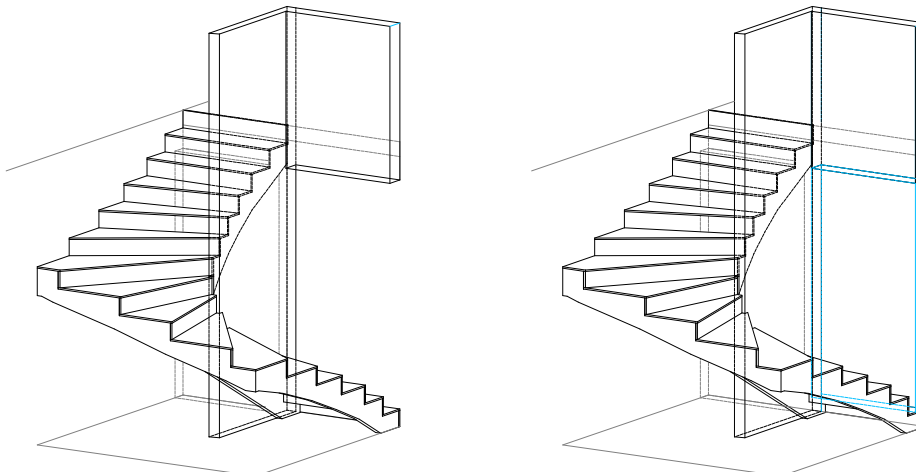
Grafik 15: Variante 2a – Fixe Stiege mit Abtrennung in Trockenbauweise unten
