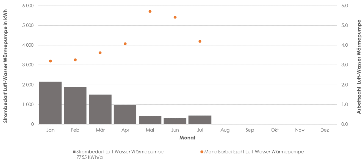
Grafik 70: Strombedarf Luft-Wasser Wärmepumpe und Monatsarbeitszahl
