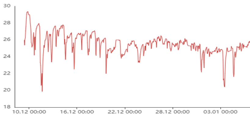
Grafik 65: Raumlufttemperatur Zimmer 2 (Top 2.5) während der Inbetriebnahmephase
